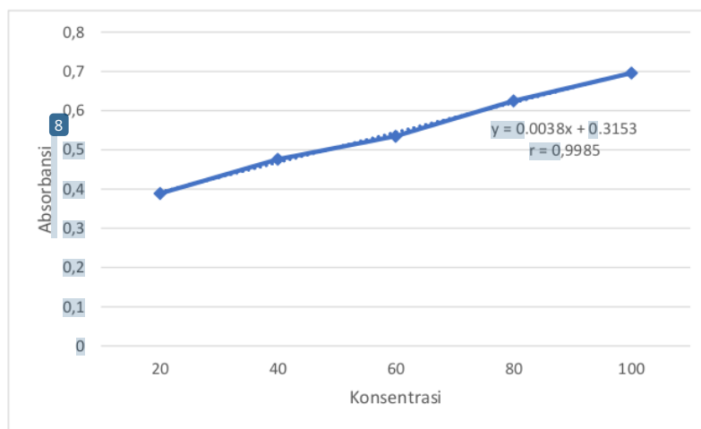
Gambar 2. Grafik Kurva Baku (Linieritas)
