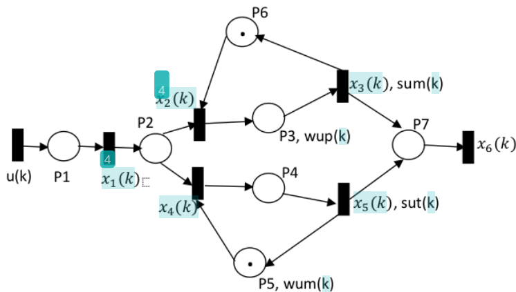
Gambar 1. Petri Net Sistem Perencanaan dan Pengadaan Obat pada Rumah Sakit
