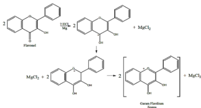
Gambar 3 Reaksi Flavonoid dengan logam Mg dan HCl
