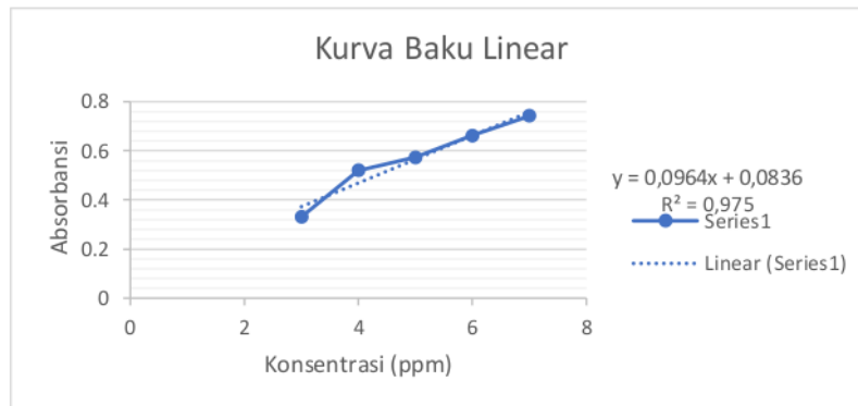
Gambar 2 Grafik Kurva Baku Linear
