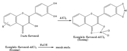
Gambar 4. Reaksi pembentukan senyawa kompleks kuersetin dengan AlCl 3
