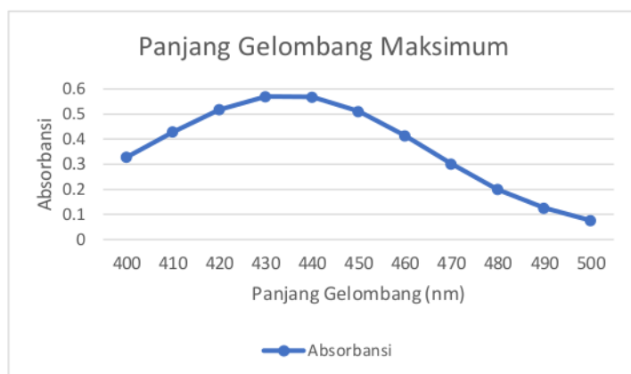
Gambar 1. Grafik Panjang Gelombang Maksimum Standar Kuersetin
