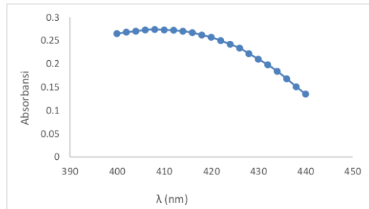
Gambar 2. Kurva \lambda_{\text{maks}} Kuersetin 70 ppm
