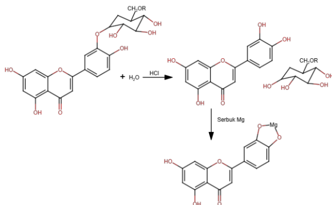
Gambar 1. Reaksi Uji Kualitatif Senyawa Flavonoid
