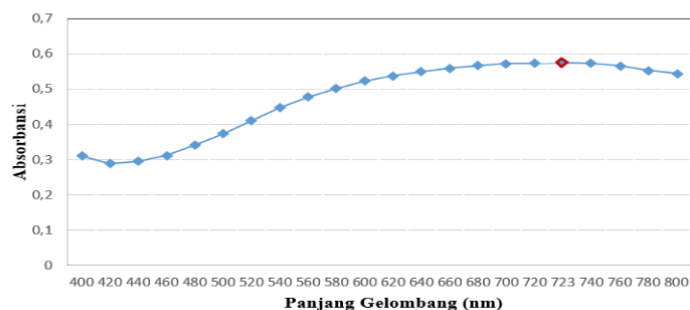
Gambar 1. Grafik Pengukuran Panjang Gelombang Maksimum
