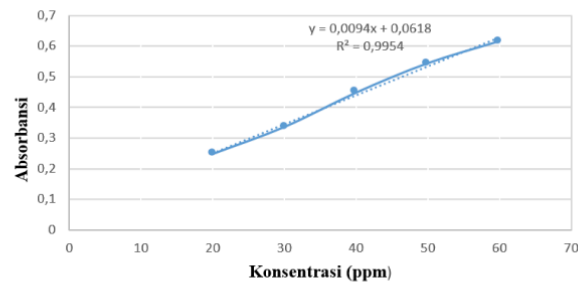
Gambar 2. Grafik Penentuan Kurva Baku
