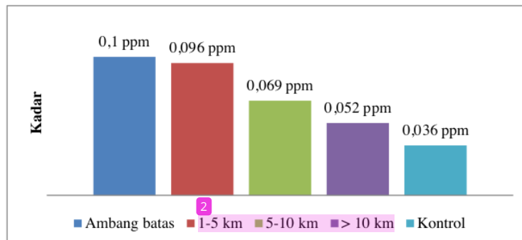
Gambar 1. Rata-rata Kadar Pb dalam Rambut pada Jarak 1-5 km, 5-10 km, > 10 km, dan Kontrol
