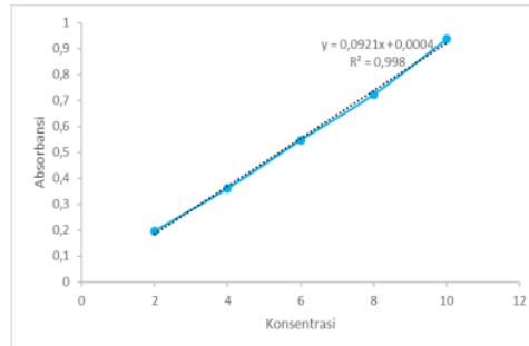
Gambar 2. Grafik Kurva Standart Vitamin C
