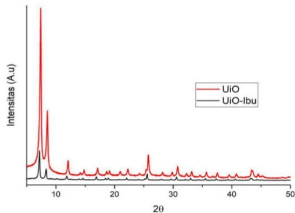
Gambar 2. Difraktogram XRD: UiO-66 (Merah); UiO-66 Loaded Ibuprofen (Hitam)
