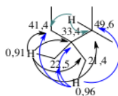
Gambar 1. Korelasi HMBC parsial 1 untuk senyawa 1
