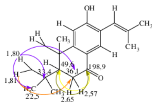
Gambar 3. Korelasi HMBC parsial 4 untuk senyawa 1
