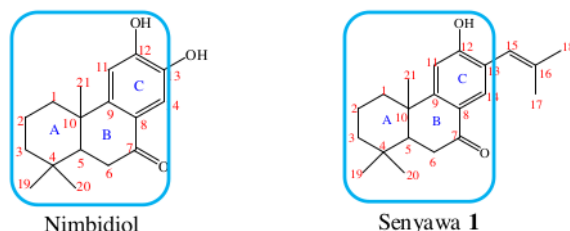
Gambar 4. Perbandingan struktur senyawa 1 dengan nimbidiol (Majumder et al. , 1987; Xie et al. , 2011)
