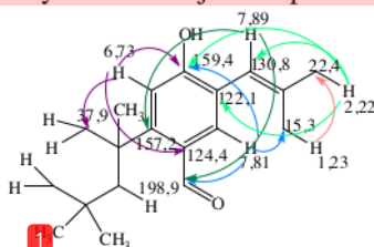
Gambar 2. Korelasi HMBC parsial 2 untuk senyawa 1
